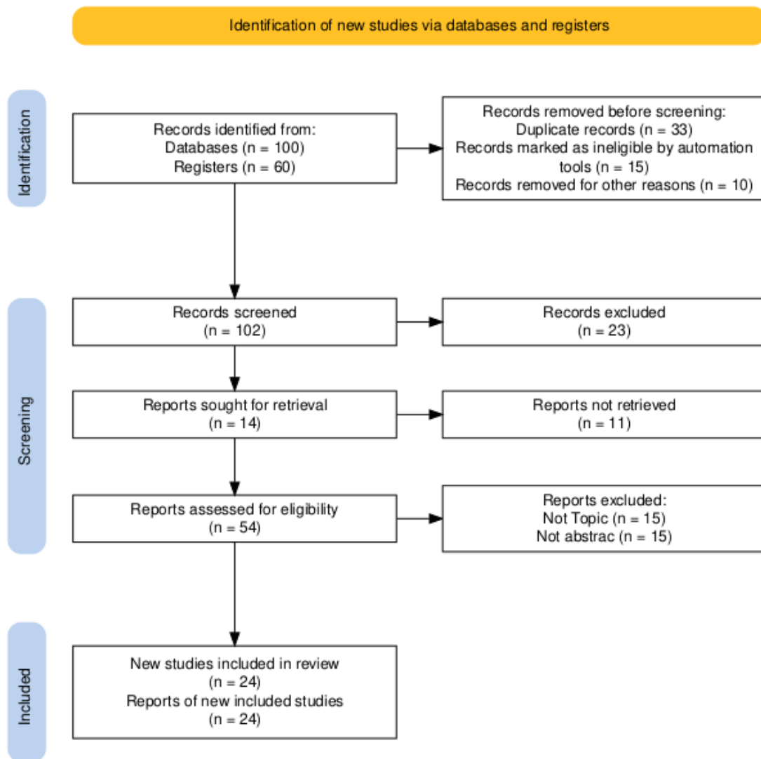
Gambar 3. Hasil PRISMA
