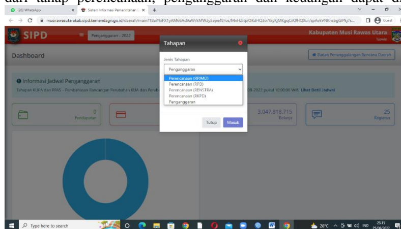
Gambar 3. tahapan SIPD
