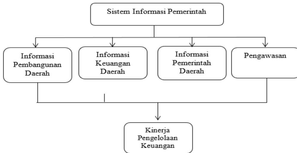
Gambar 1. Kerangka Berpikir
