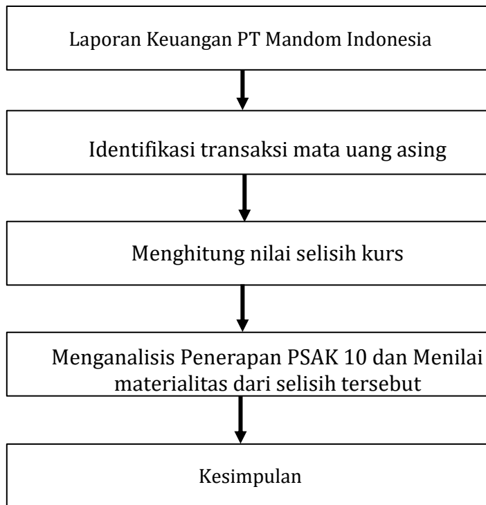
Gambar 2. Kerangka Konseptual
